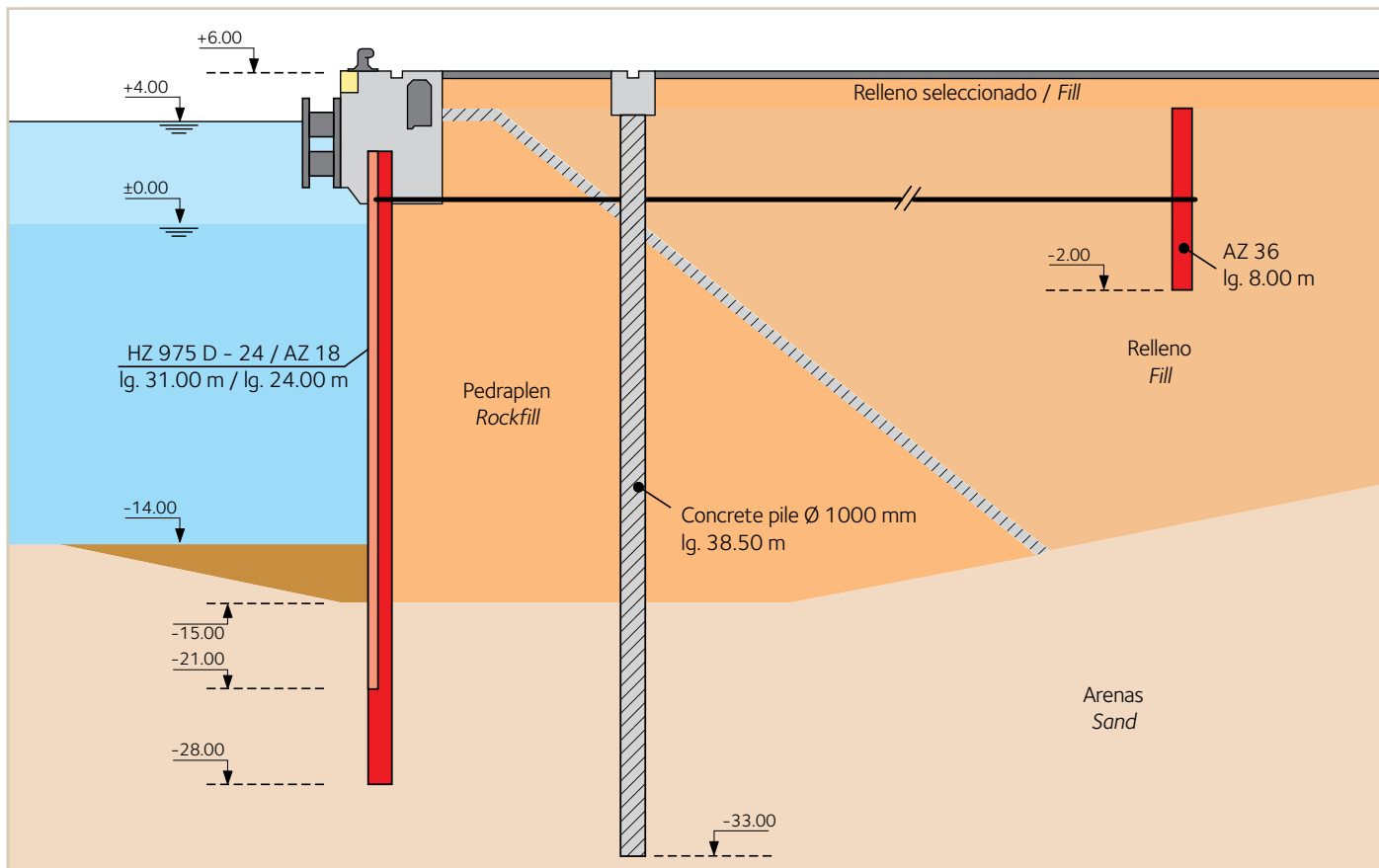
Для строительства причальной стенки высотой 20 м использовали комбинированную шпунтовую систему типа HZ/AZ.
