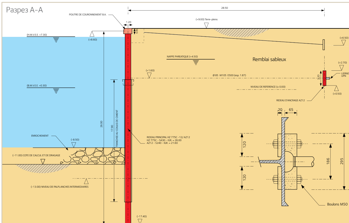
Поперечный разрез шпунтовой стенки вдоль борта паром (HZ775C-12/AZ12).
