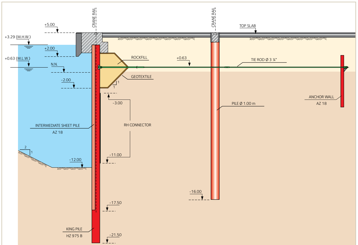
В основе современного терминала шпунтовая система HZ/AZ с анкерной системой.
