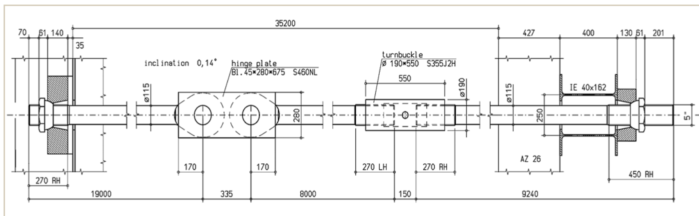
Для оптимизации транспортировки стальные анкерные тяги поставлялись тремя отдельными звеньями.
