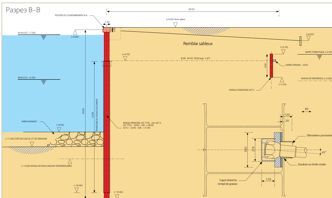
Поперечный разрез шпунтовой стенки, параллельной носовой части паром (HZ775C-24/AZ12).
